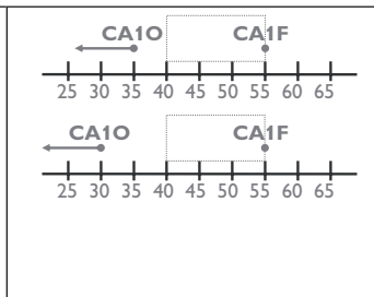
Desplazamiento automático de CA1F hacia abajo si, antes del ajuste, CA1O se ha ajustado en el rango (CA1F - 15K)
