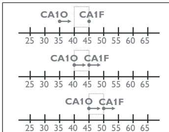
Desplazamiento automático de CA1F hacia arriba cuando CA1O alcanza el límite (CA1F - 5K)
